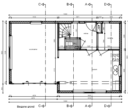
Begane grond 1:100
