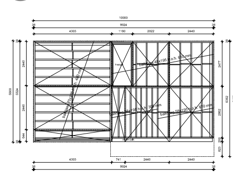
principe verdiepingvloer
