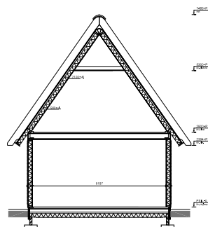
Doorsnede C-C
