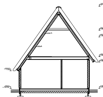
Doorsnede D-D
