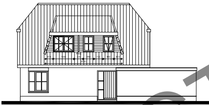
Linker zijgevel
