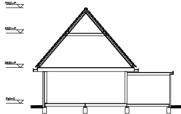
Doorsnede
